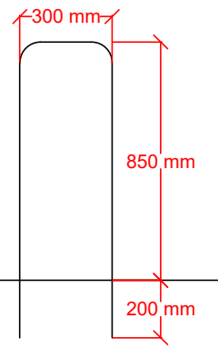
PERIAATEKUVA UPPOASENNUKSESTA
